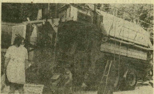
A makóiak egyik legújabb gyártmánya, a rendfelszedő borsócséplő gép
